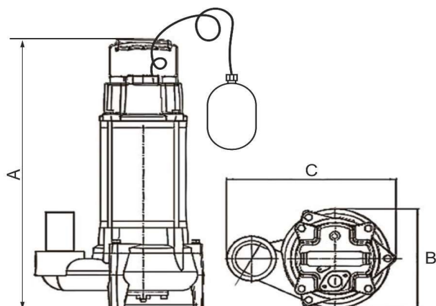
Габаритные размеры
