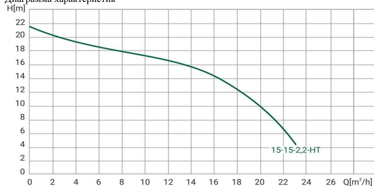
Диаграмма характеристик
